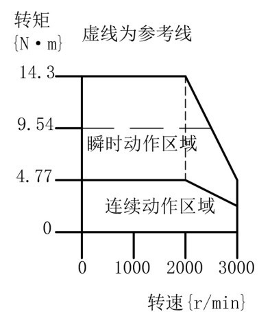
动态转矩特性： 电源电压 (AC:220V)
