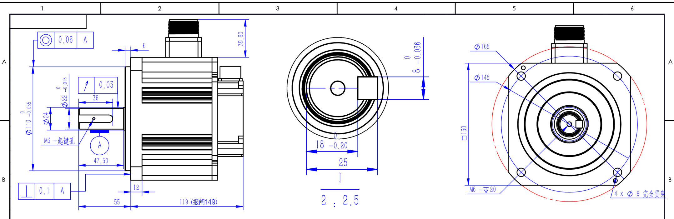
电机技术规格 Motor specifications
