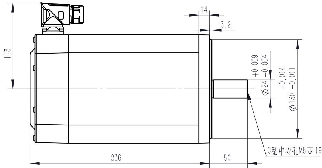
电机技术规格 Motor specifications
