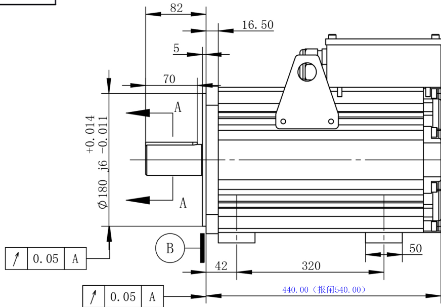
电机技术规格 Motor specifications
