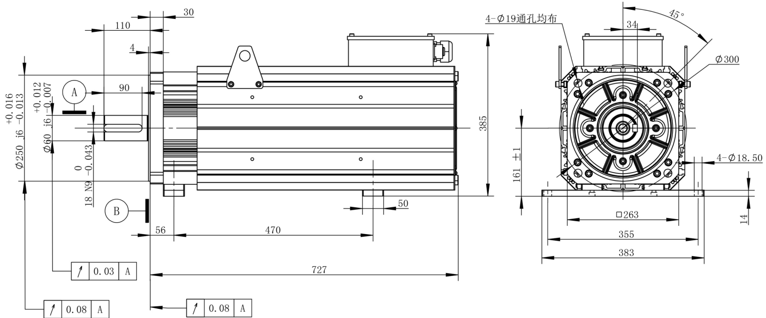
电机技术规格 Motor specifications
