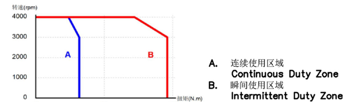
转速-转矩 特性曲线
