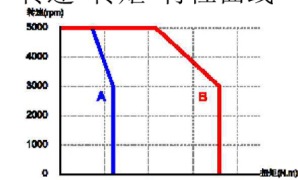
A. 连续使用区域 Continuous Duty Zone B. 瞬间使用区域 Intermittent Duty Zone
